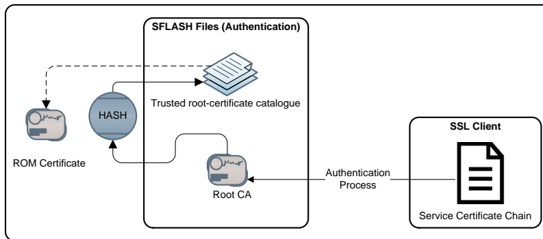
图 7. 证书文件及其与受信任根证书目录之间的关系
