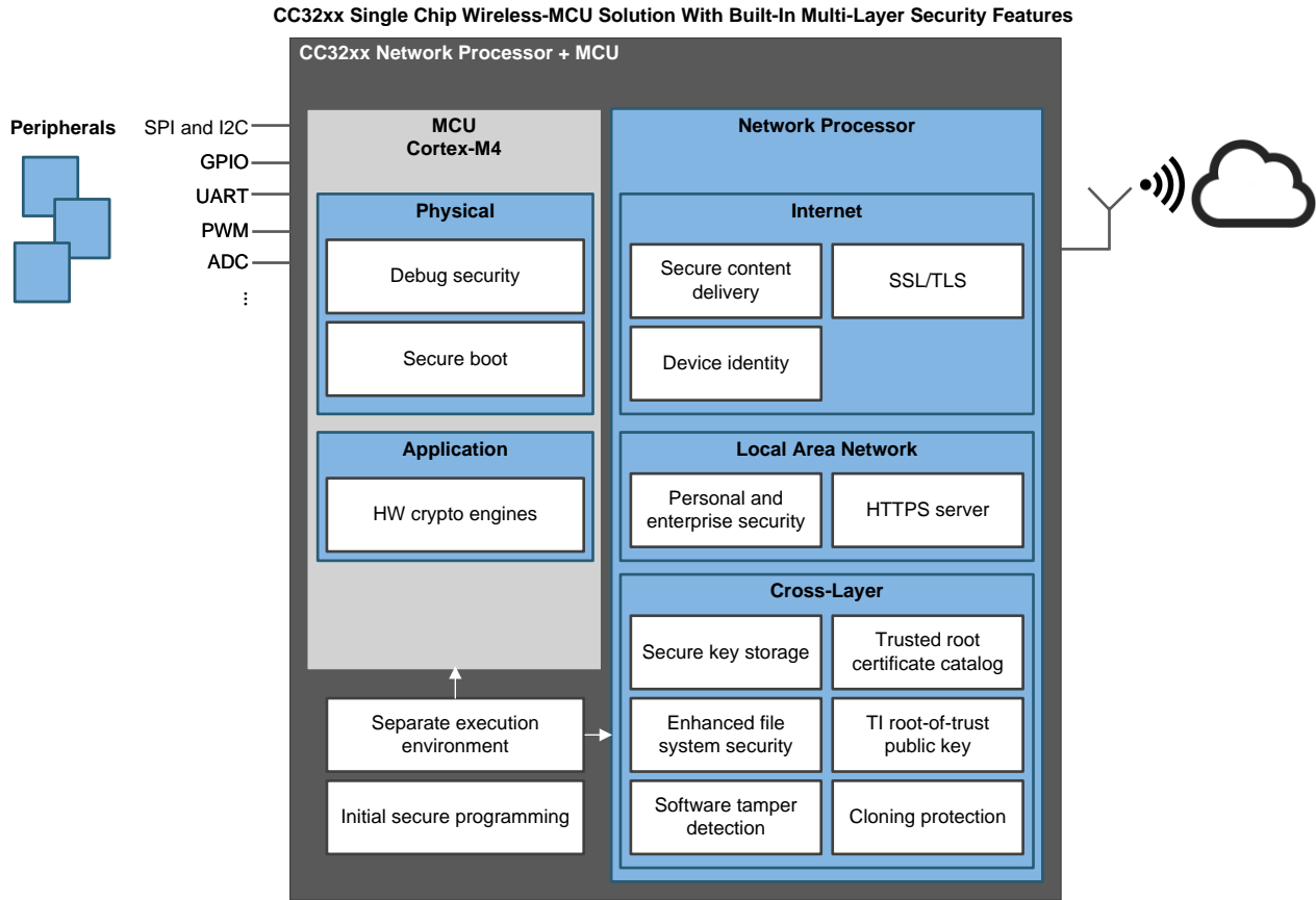
图 3. CC3220 安全 功能
