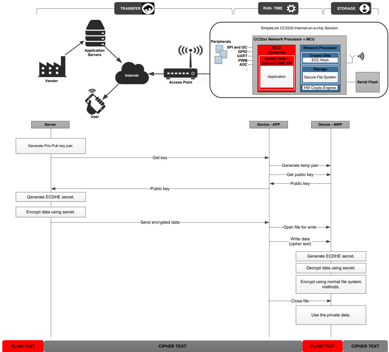
图 9. 安全内容交付 - 过程 说明
