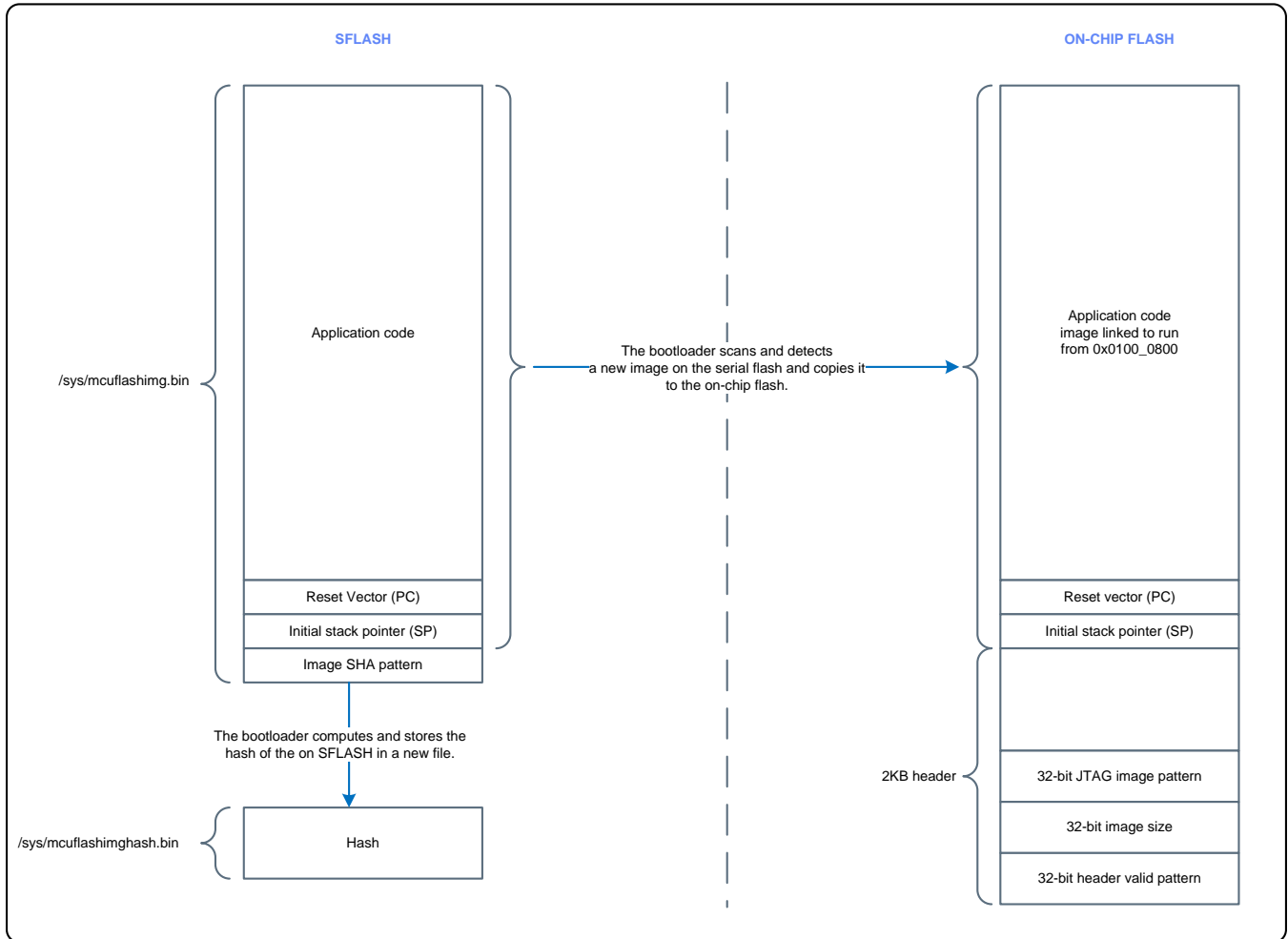
图 11. 片上闪存编程和更新
