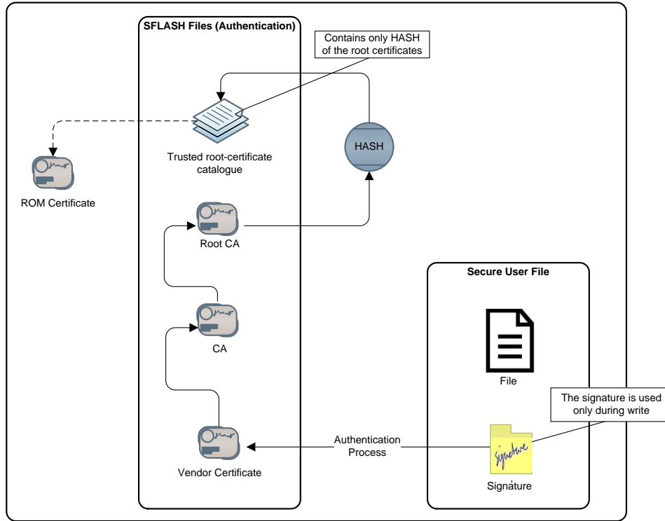
图 8. 验证文件签名
