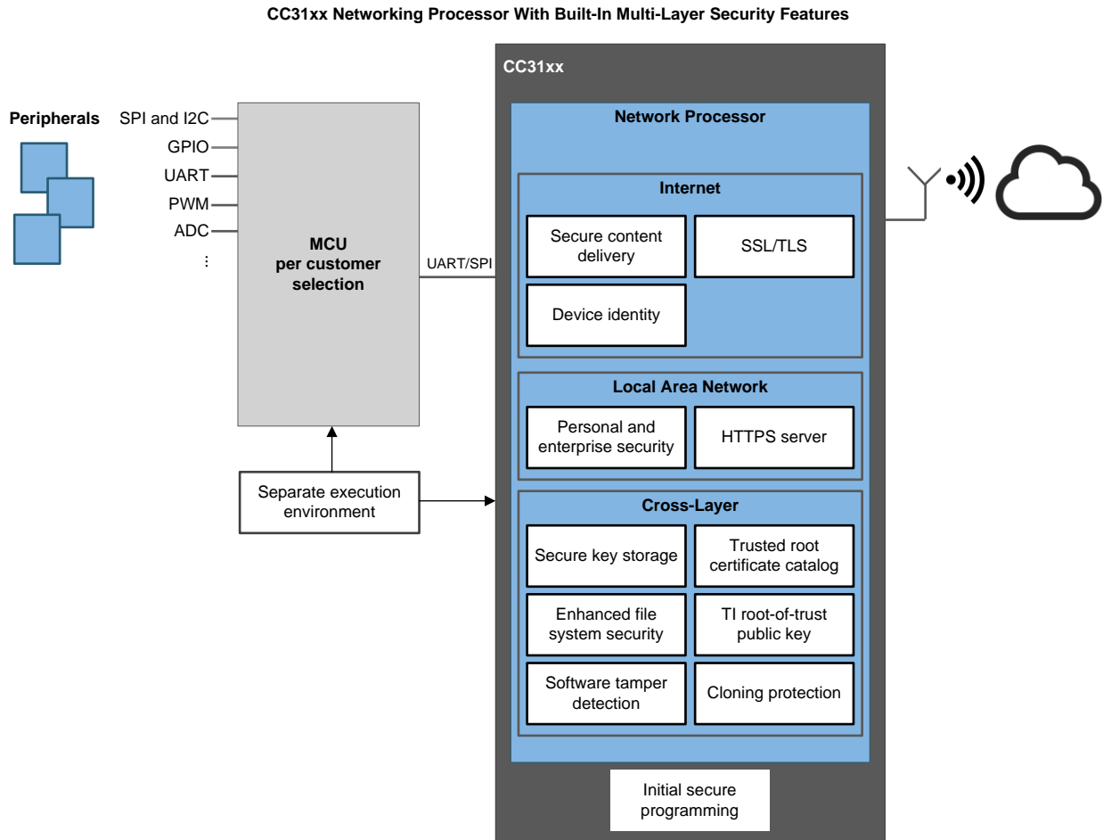
图 4. CC3120 安全功能
