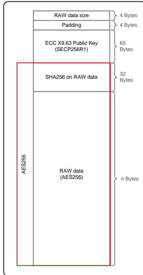
图 10. 安全内容交付 - 文件格式
