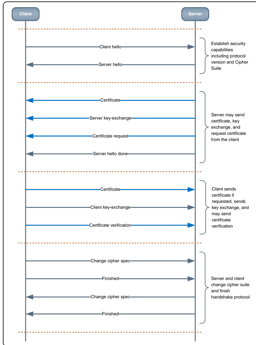
图 6. SSL 握手
