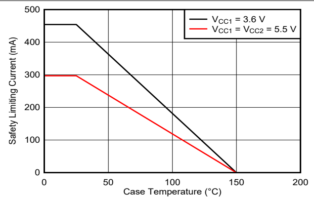
图 6-2. 符合 VDE 的 DW-16 热降额曲线
