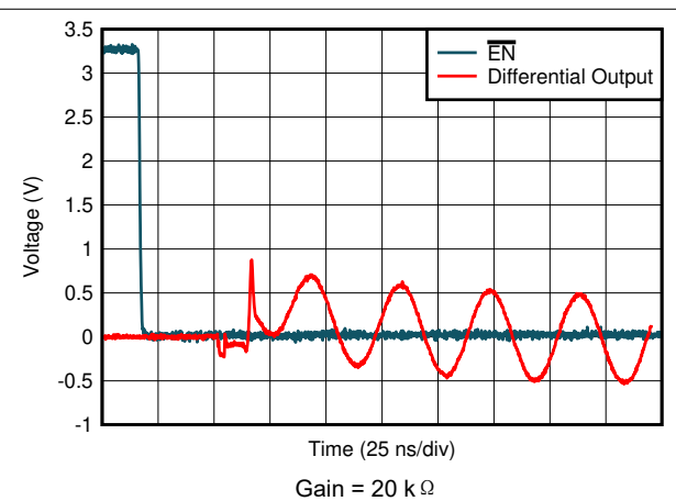
图 6-24. Turn-On Time
