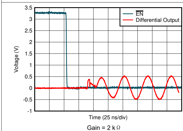
图 6-23. Turn-On Time
