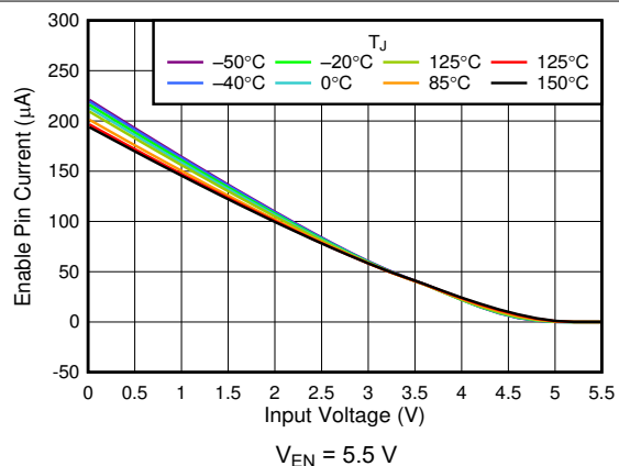
图 5-16. I_{EN} vs V_{IN}
