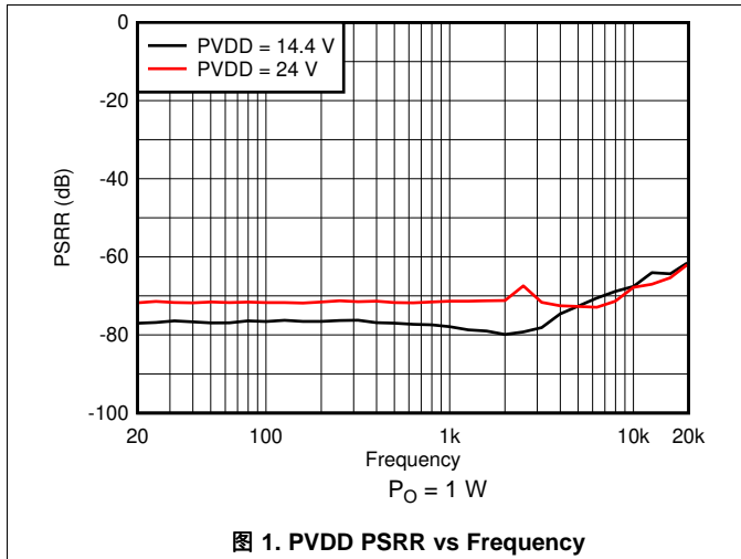
图 1. PVDD PSRR vs Frequency
