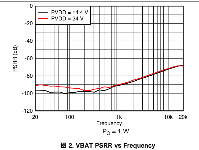
图 2. VBAT PSRR vs Frequency
