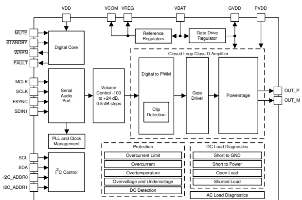
功能方框图
