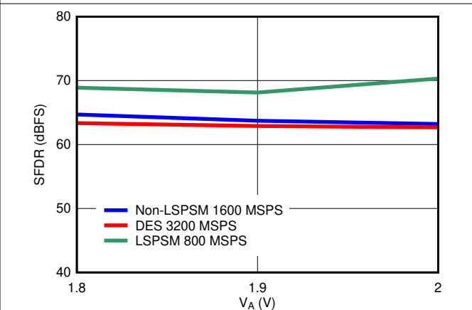
图 6-28. SFDR vs Supply Voltage
