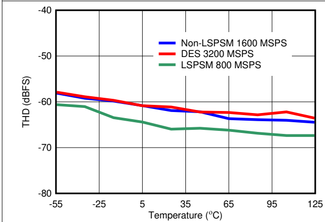
图 6-25. THD vs Temperature
