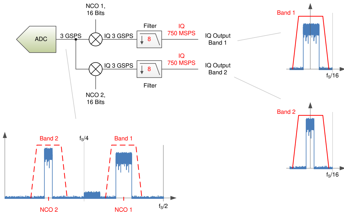
图 8-17. Dual-Band Example
