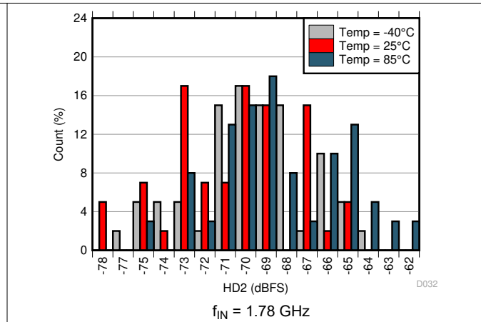
图 6-56. HD2 Histogram at AVDD19 = 1.9 V
