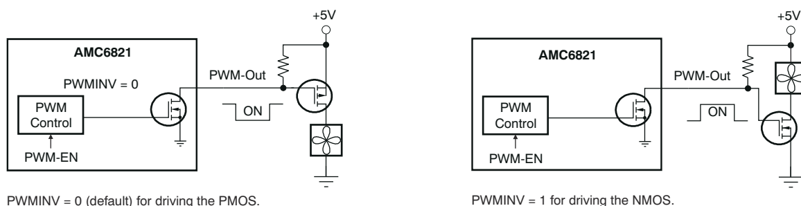
图 8-5. PWM Output
