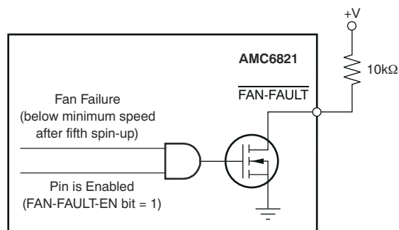
图 8-11. \overline{\text{FAN-FAULT}} Pin
