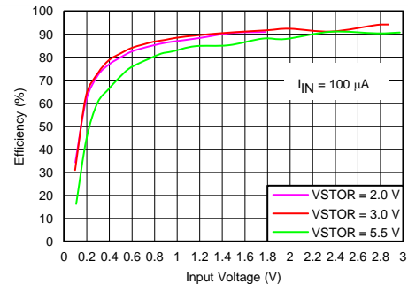
充电器效率
