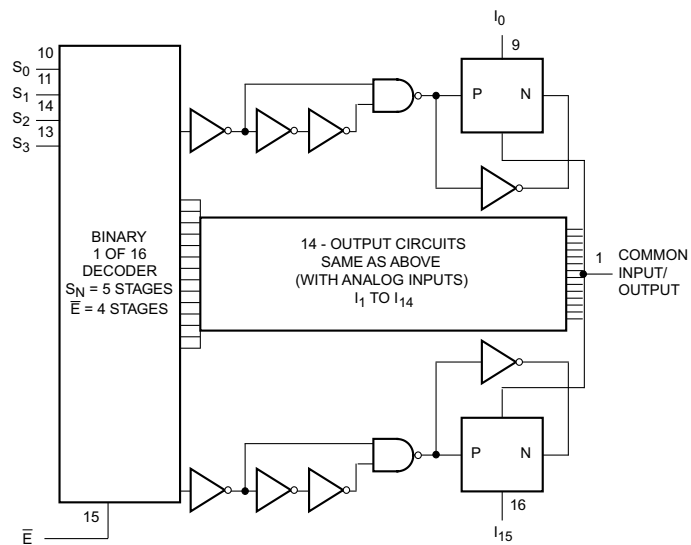
功能方框图
