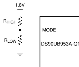
图 7-7. MODE Configuration
