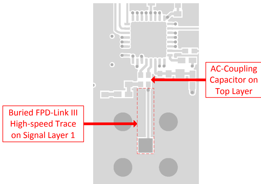
图 10-1. DS90UB953A-Q1 Serializer DOUT+ Trace Layout
