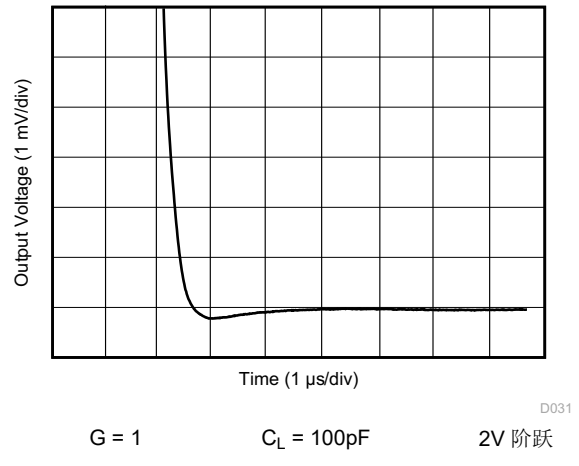
图 6-25. 大信号稳定时间 (负)
