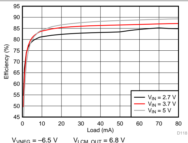
图 204. VNEG Efficiency
