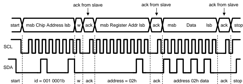
图 46. Register Write Format
