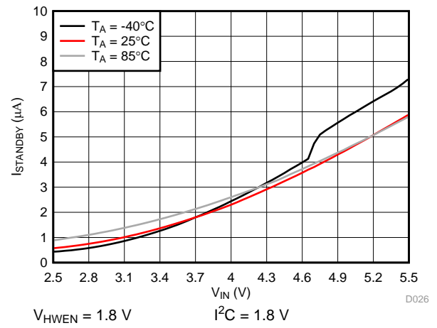
图 29. I_q Standby
