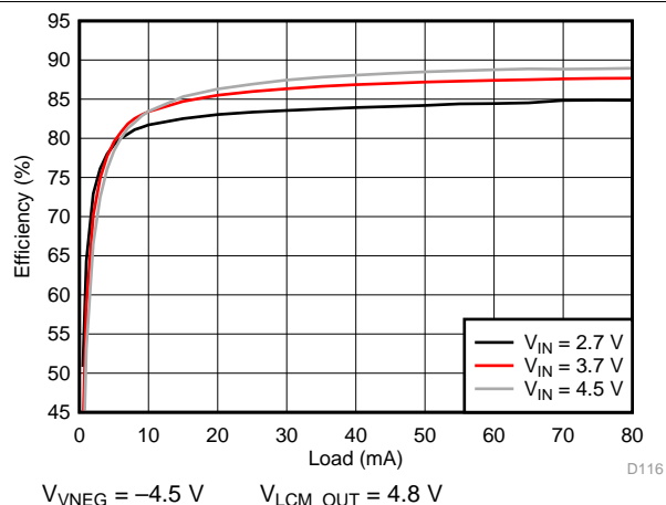
图 202. VNEG Efficiency
