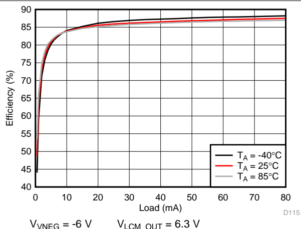
图 201. VNEG Efficiency
