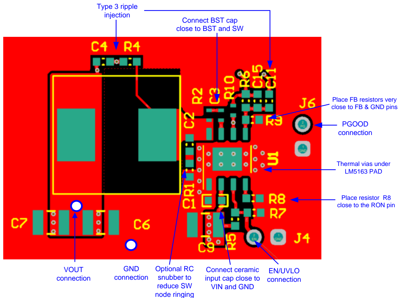
图 28. LM5163-Q1 Single-Sided PCB Layout Example
