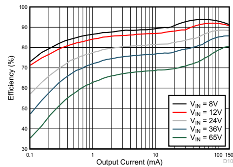
图 6-2. Converter Efficiency: 5 V, 150 mA, COT
