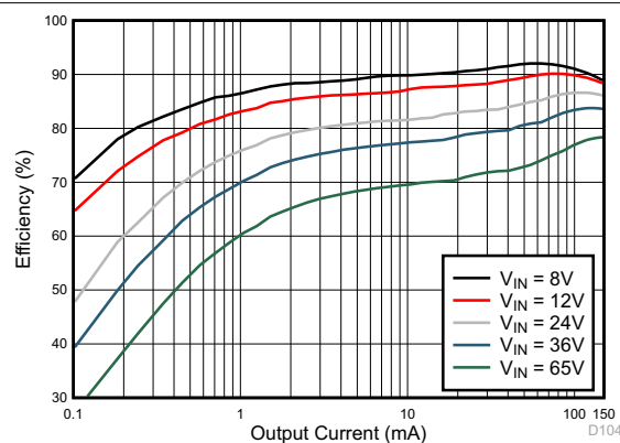
图 8-27. Efficiency
