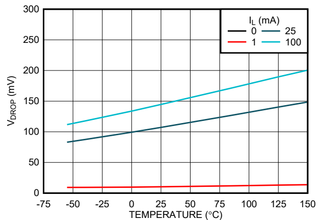
压降电压与温度间的关系 (新芯片)
