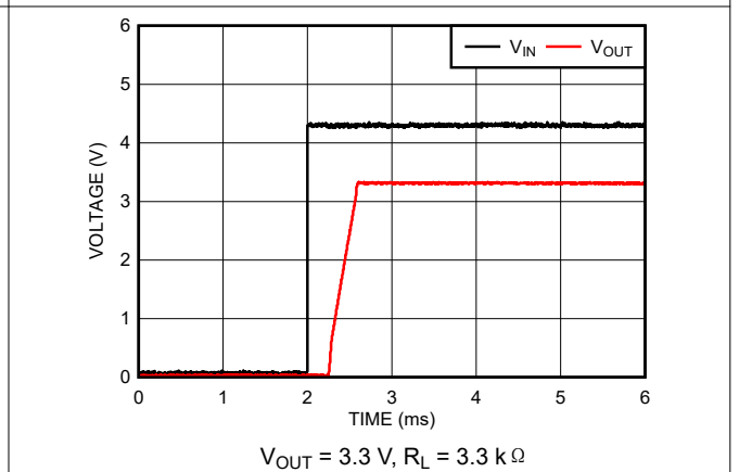
图 7-10. Turn-on Waveform (New Chip)
