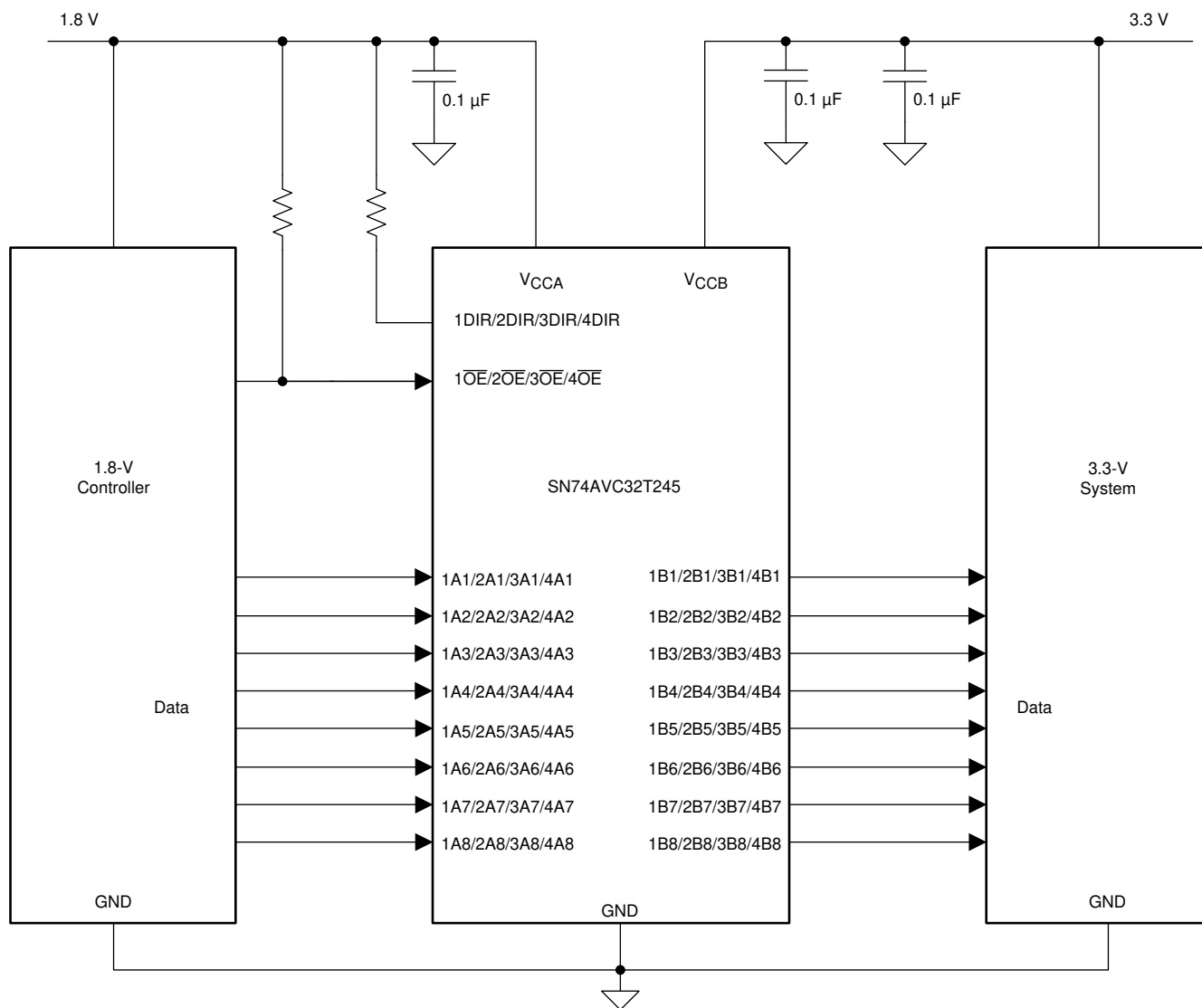
图 10-1. 应用原理图
