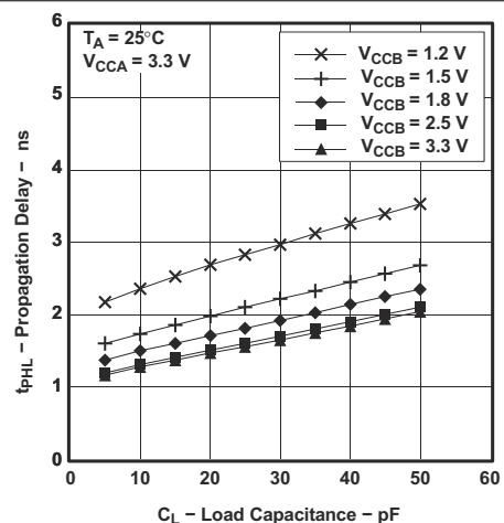
图 7-10. 传播延迟与负载电容间的关系
