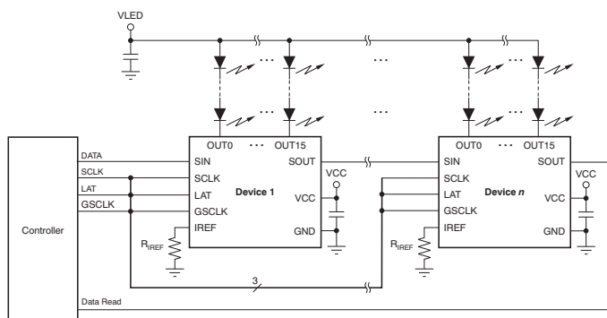
典型应用电路（多菊花链 TLC5948As）
