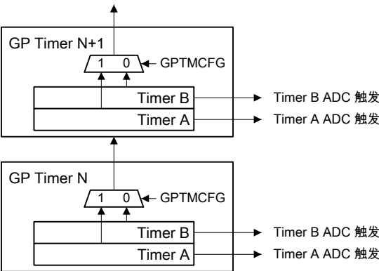
图 11-9. 定时器菊花链
