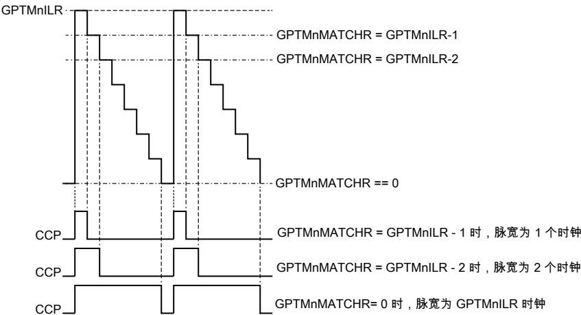
图 11-8. CCP 输出，GPTMTnILR > GPTMTnMATCHR
