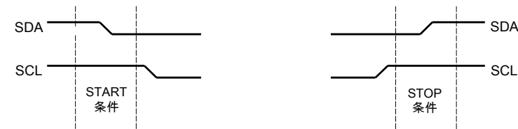
图 16-3. START 和 STOP 条件
