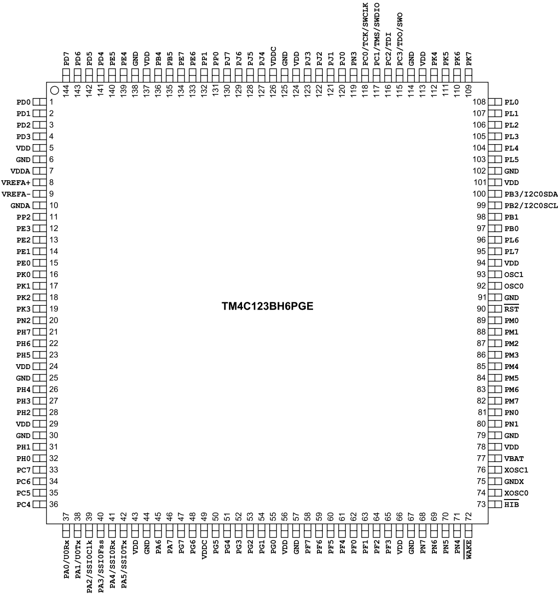
图 21-1. 144 管脚 LQFP 封装管脚图
