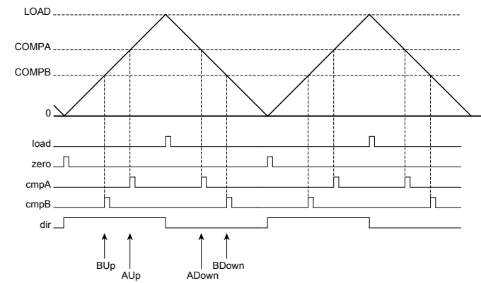
图 19-4. PWM先递增后递减计数模式
