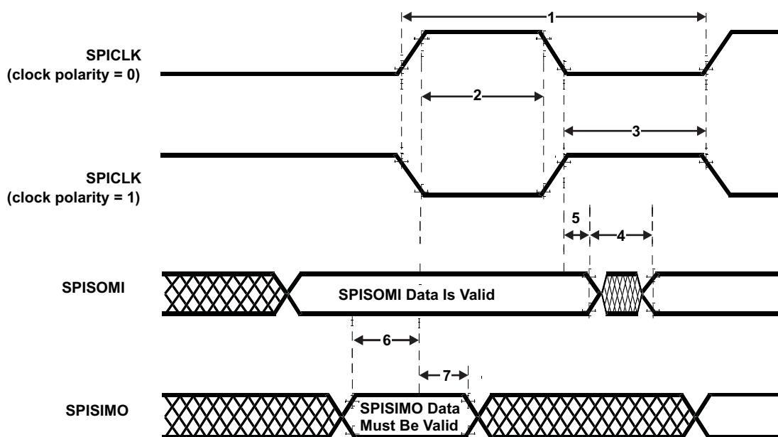
图 6-12. SPI 受控模式外部时序 (时钟相位 = 1)
