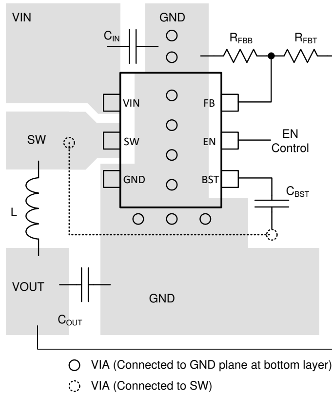
图 11-1. TPS562202 布局
