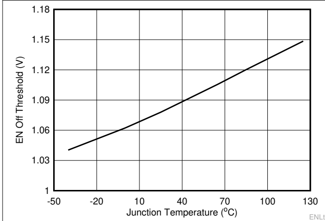
图 7-3. EN 关断阈值电压与结温间的关系
