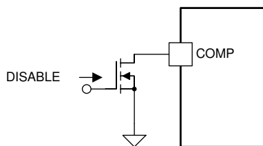
图 8-7. Disable Circuit
