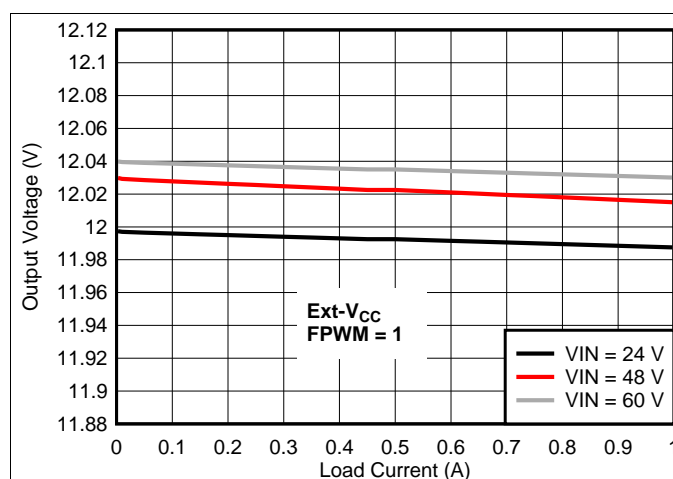
图 26. Load Regulation
