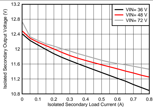
图 35. Load Regulation
