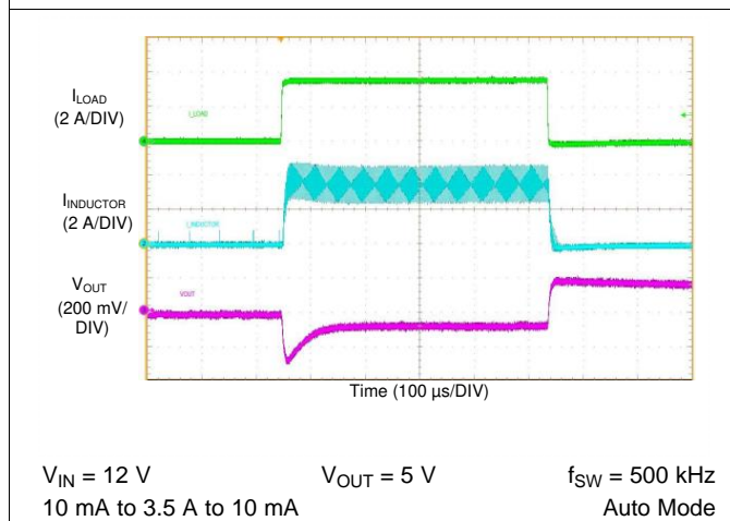
图 75. LM76003-Q1 Load Transient
