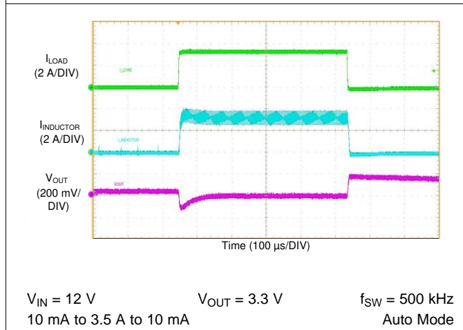
图 73. LM76003-Q1 Load Transient
