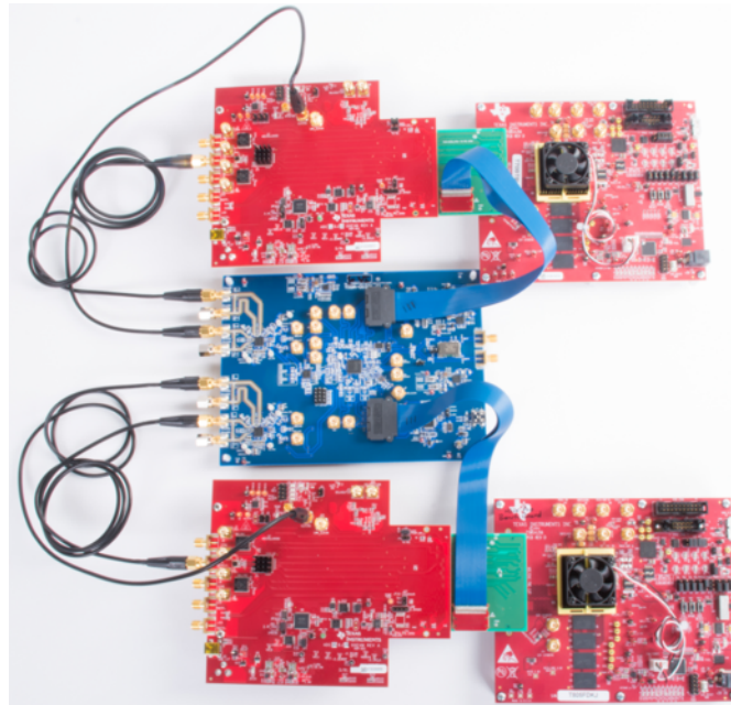
图 3. Test Setup
