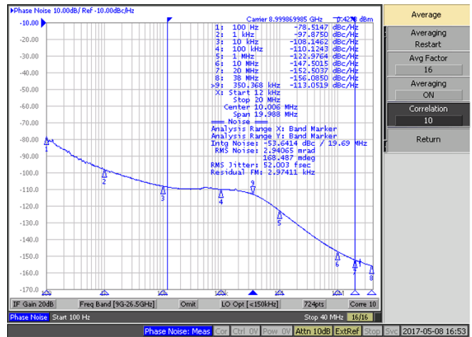
图 11. Phase Noise at 9 GHz
