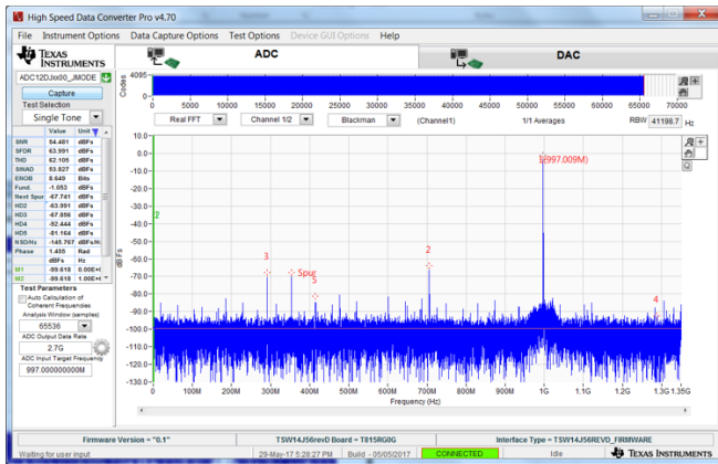
图 14. Spectrum at 997-MHz Input
