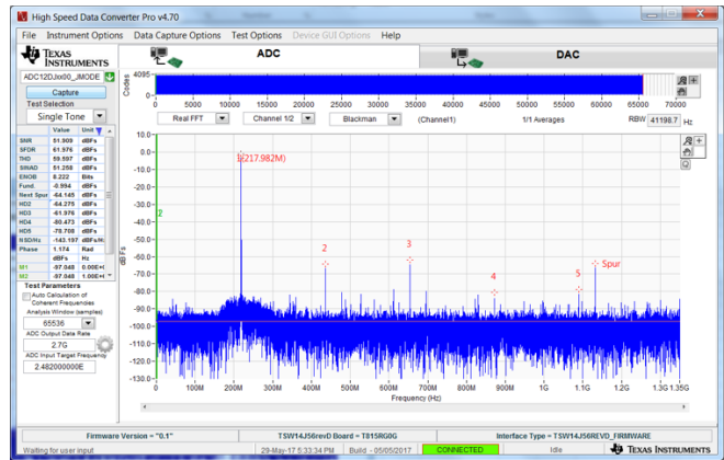
图 15. Spectrum at 2482-MHz Input
