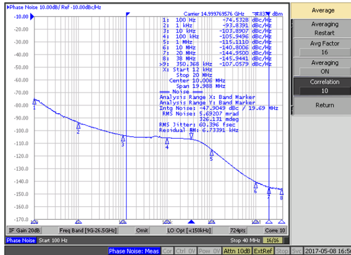
图 12. Phase Noise at 15 GHz
