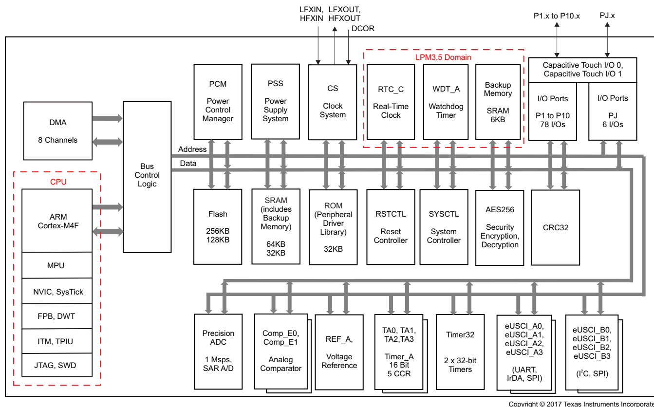
图 3. MSP432P401R Block Diagram
