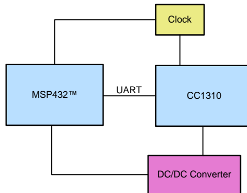
图 2. TIDA-01547 System Block Diagram
