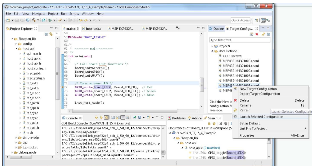
图 24. Launch CCS™ Target Configuration
