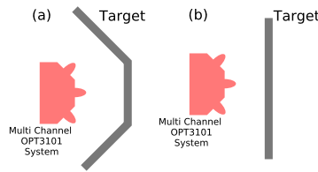
图 9. 相位偏移校准设置
