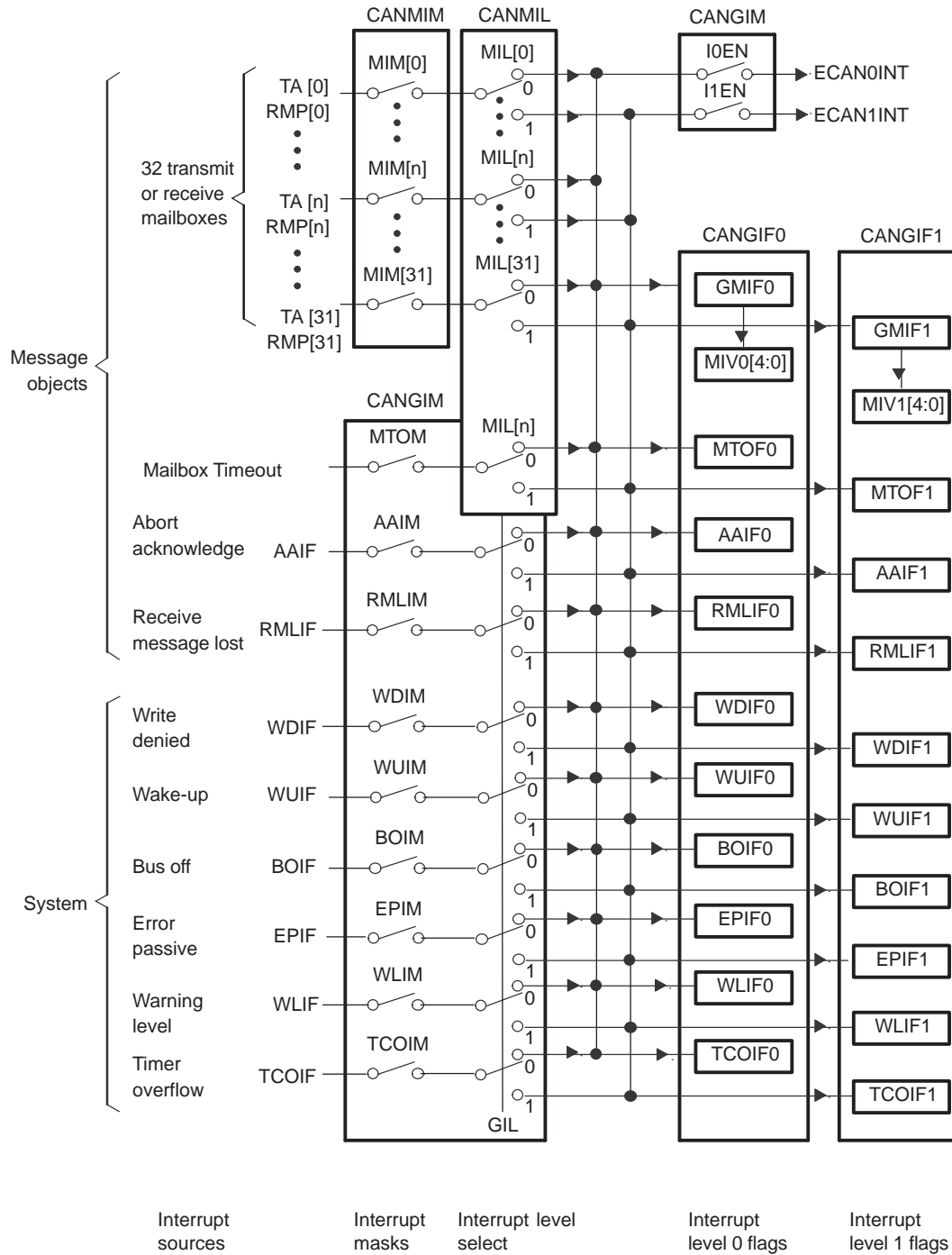
图 43. 中断方案
