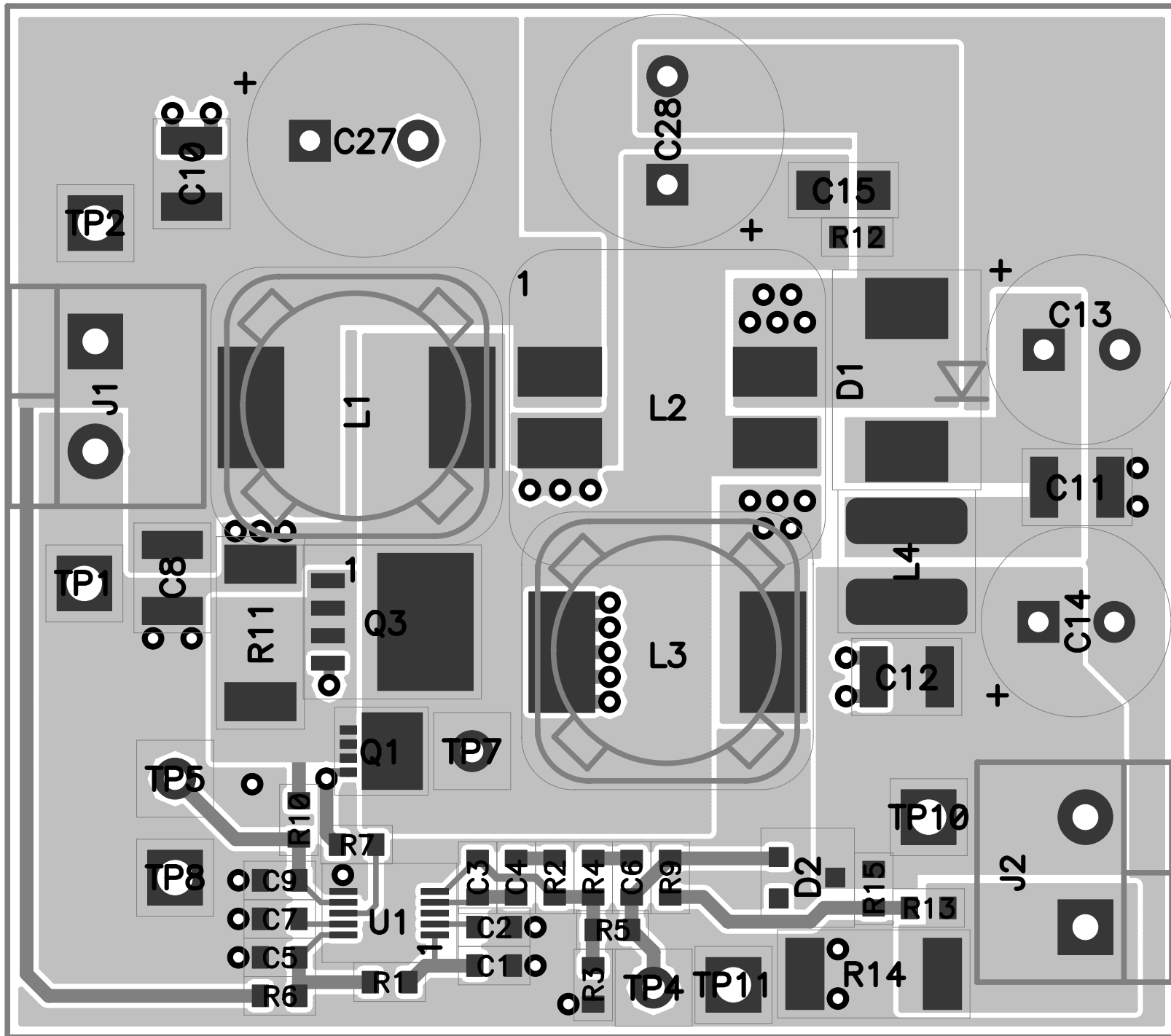
LAYER 1-TOP
