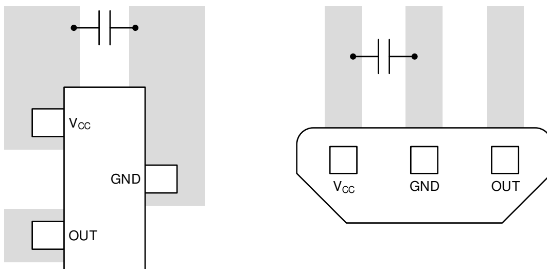
図 7-5. Layout Examples
