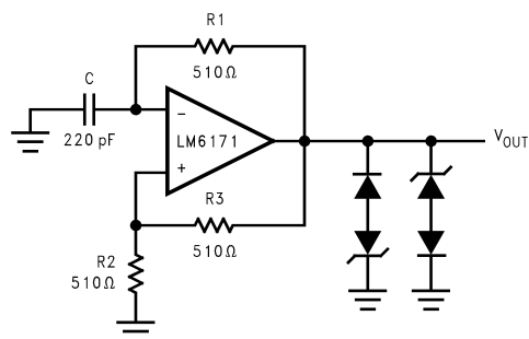
図 7-8. Multivibrator
