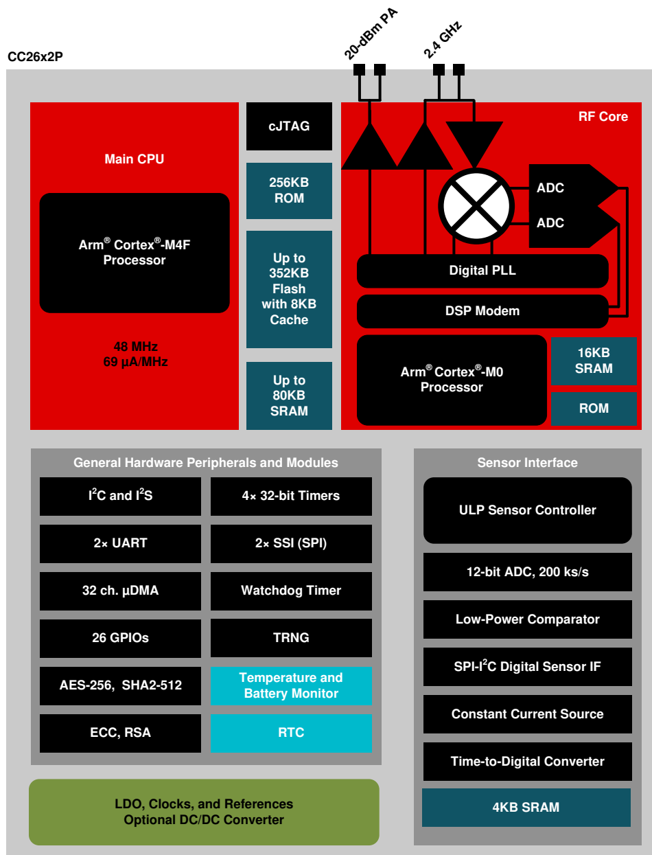
図 4-1. CC2652P Block Diagram
