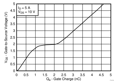
ゲート電荷
