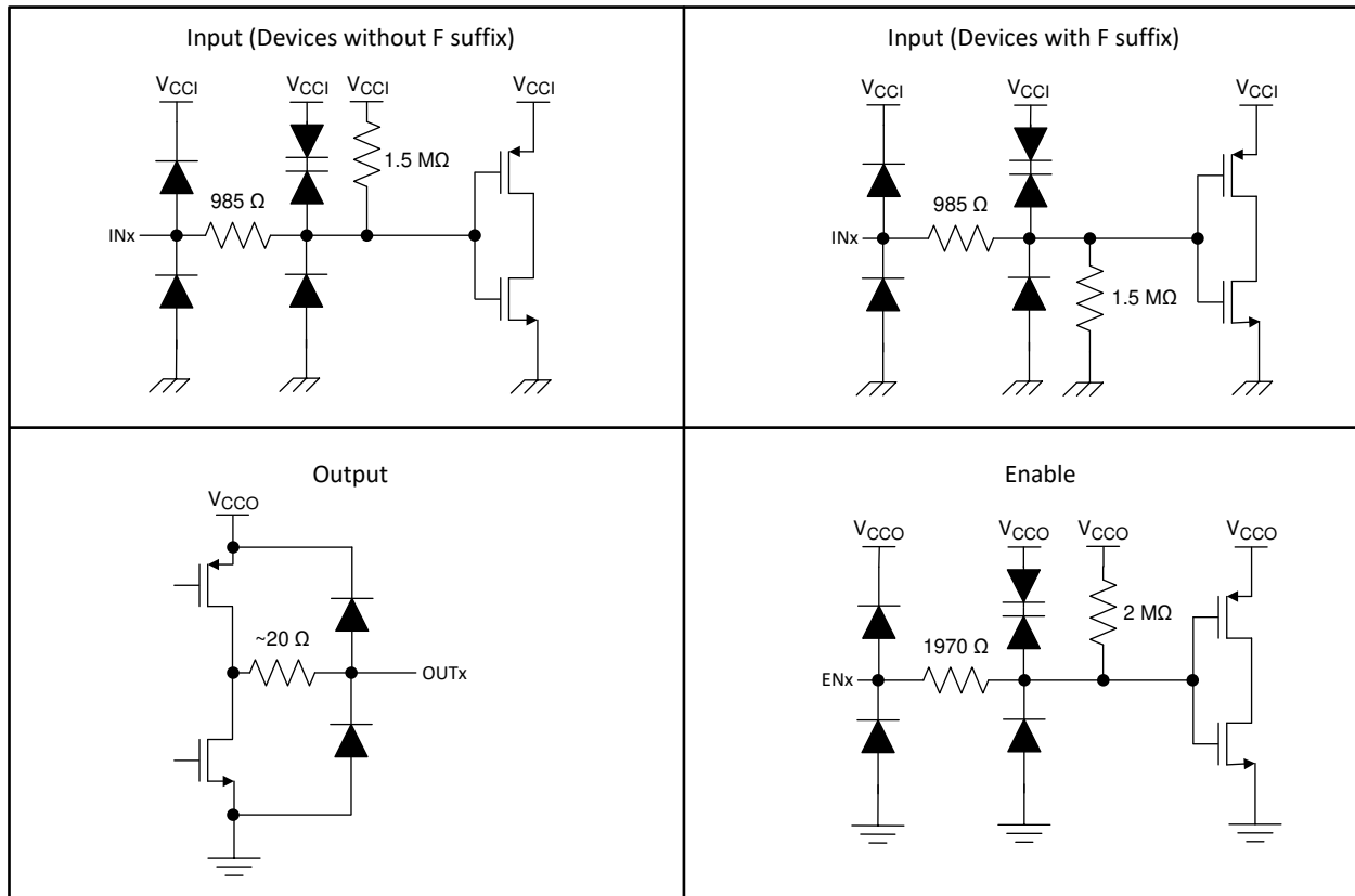
図 8-3. Device I/O Schematics
