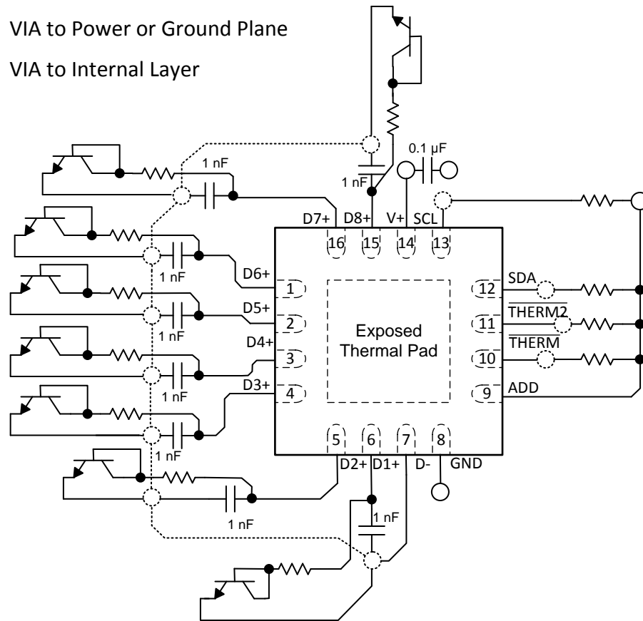
⊗ 28. TMP468 RGT Package Layout Example
