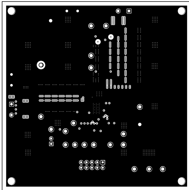
8-11. EVM Inner Layer 1
