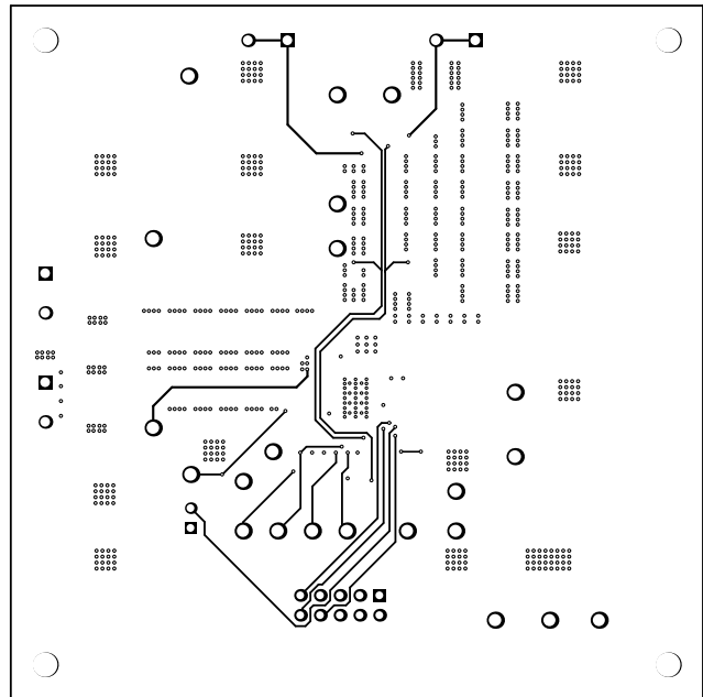
8-12. EVM Inner Layer 2
