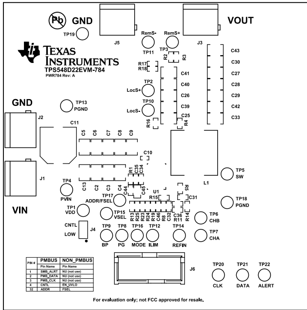
8-9. EVM Top View
