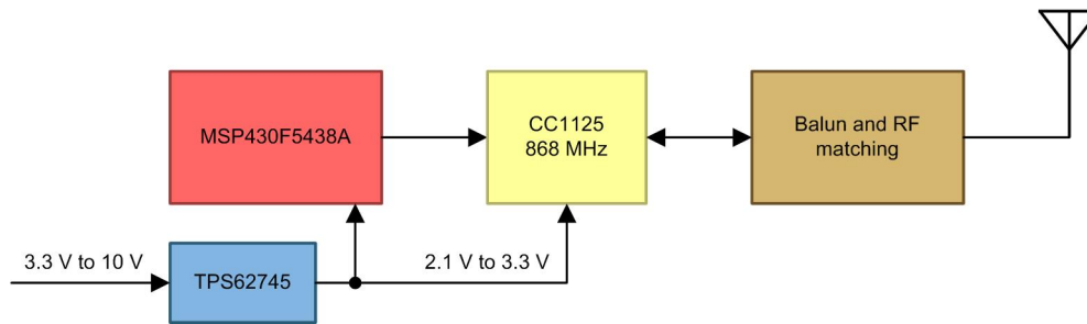
図 4. TIDC-DSSS868WMBUS-DC Block Diagram
