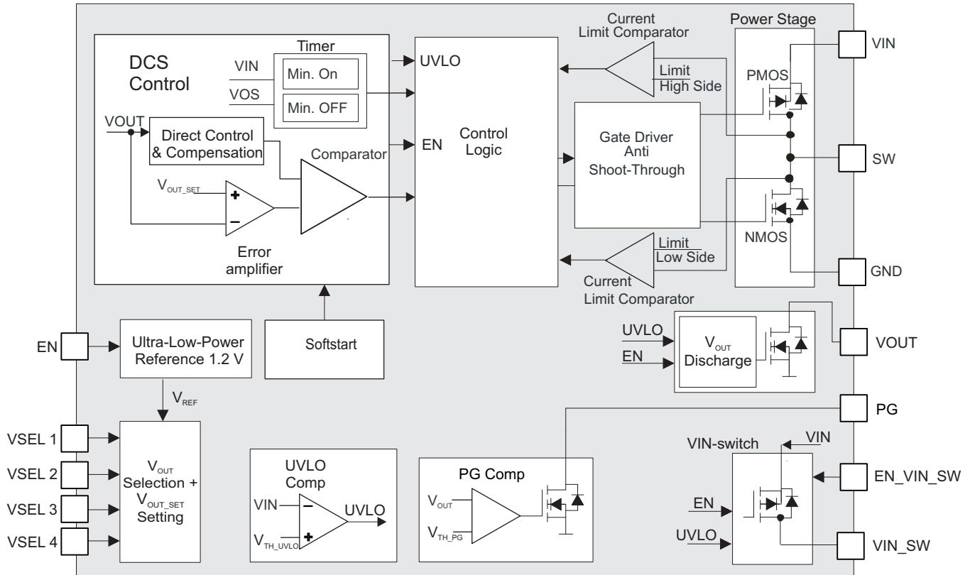
図 3. TPS62745 Block Diagram
