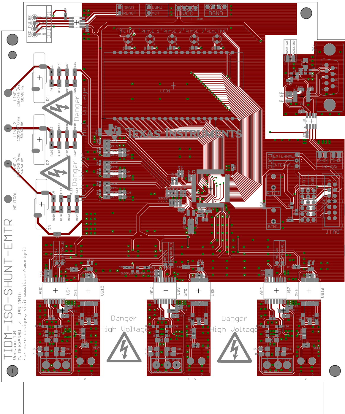
TIDA-00601 TOP LAYER
