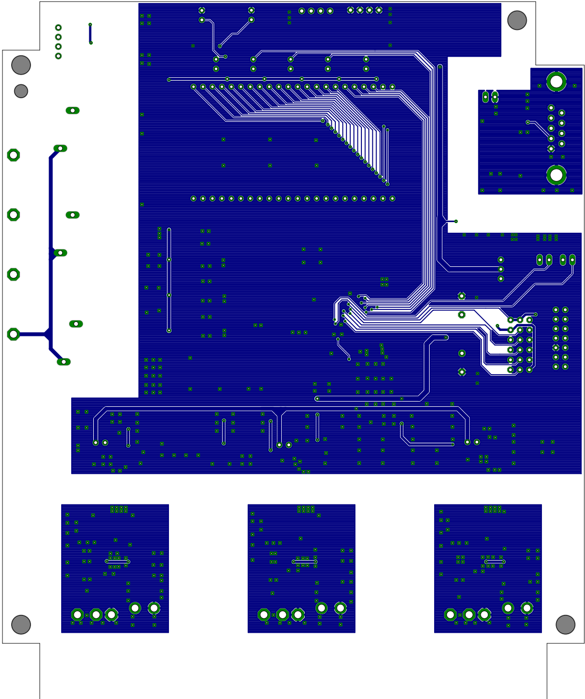
TIDA-00601 BOTTOM LAYER
