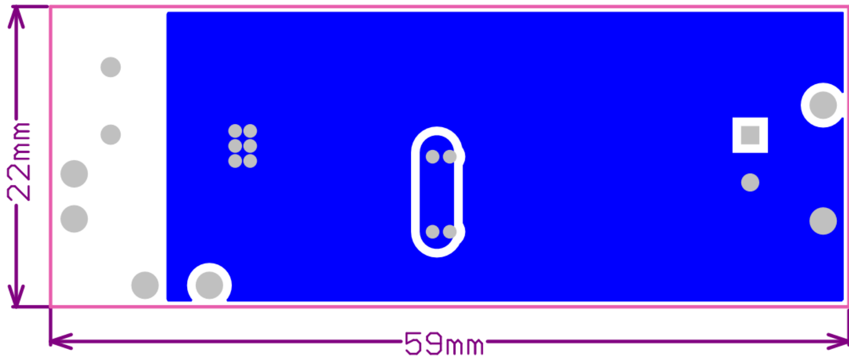
PMP30364 Layer Plot Bottom
