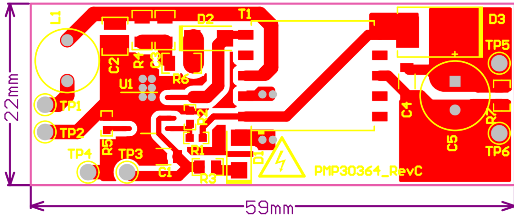
PMP30364 Layer Plot Top
