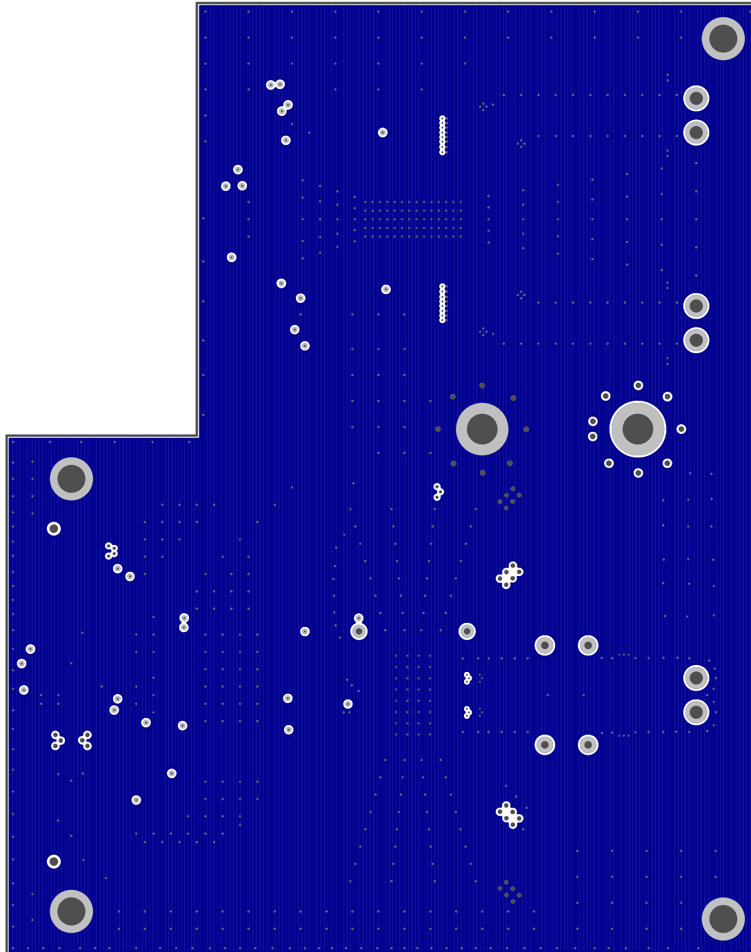
COPPER LAYER 2
