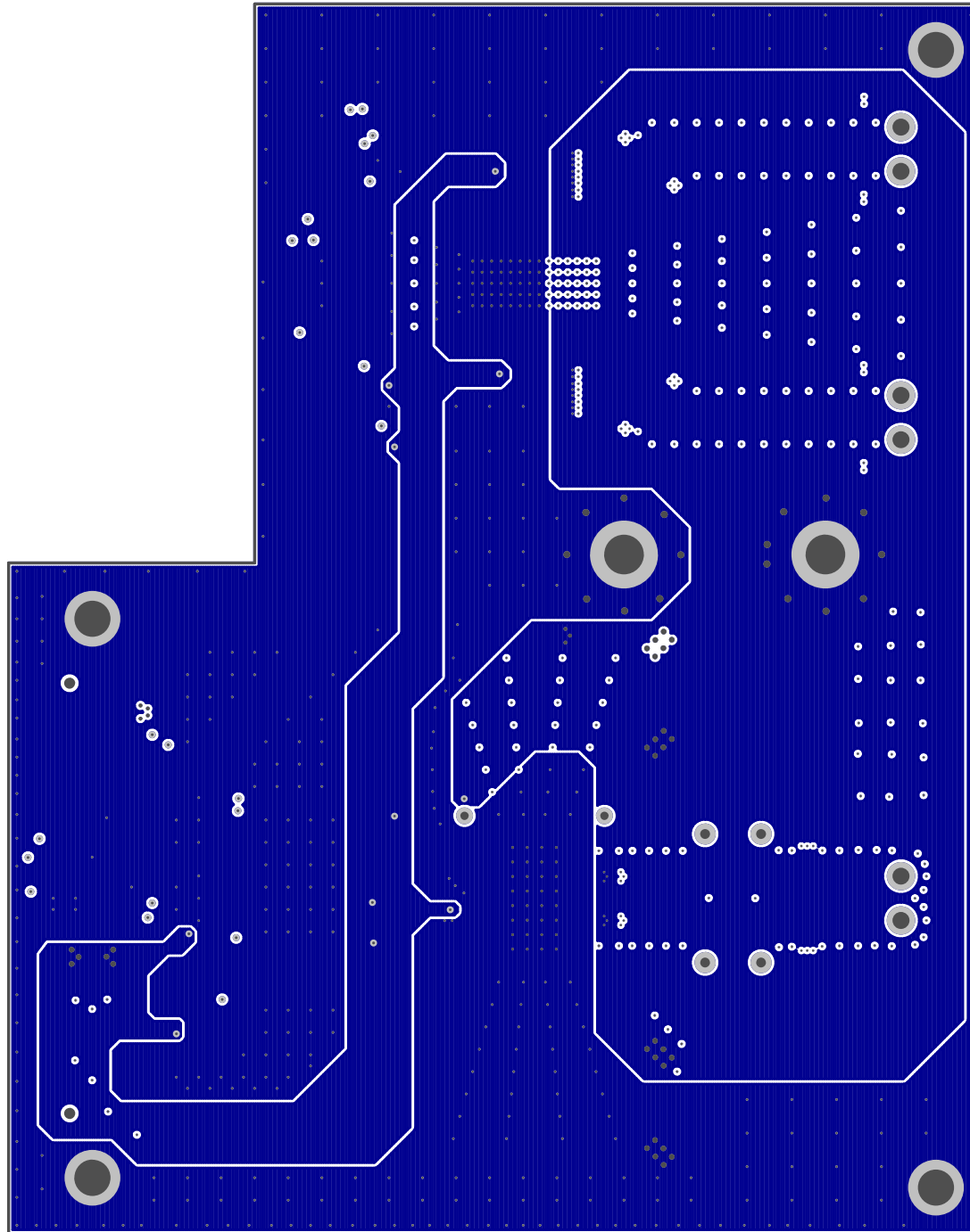
COPPER LAYER 3
