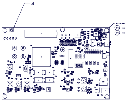
TOP SIDE
