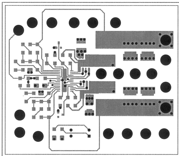
Figure 26. Top Layer
