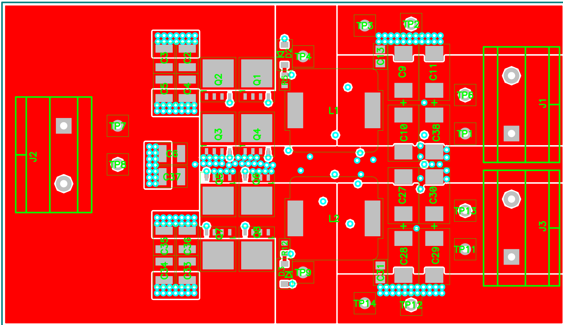
PMP3199 REV A LAYER 1-TOP
