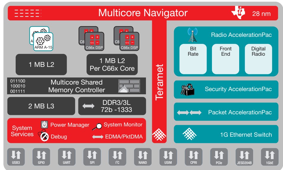
▲ KeyStone II-based TCI6631K2L SoC
