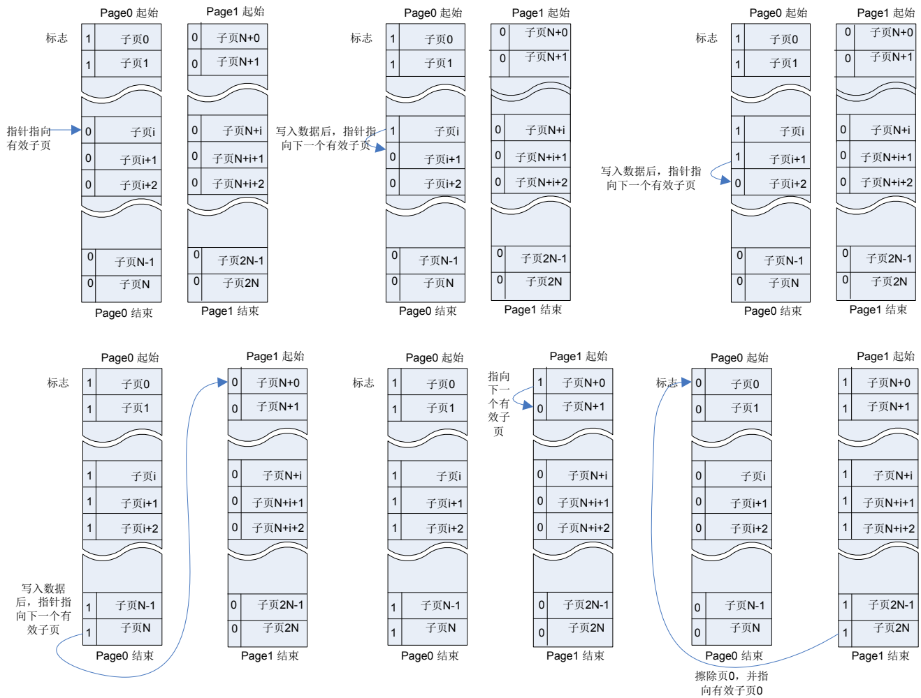
图三 使用子页的方式模拟 EEPROM 存储单元
