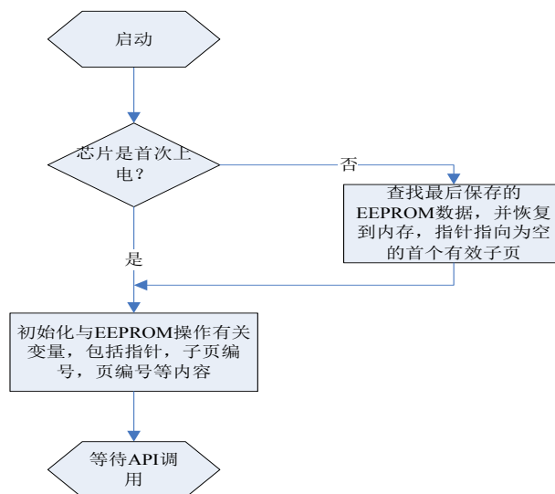
图四 初始化流程图
