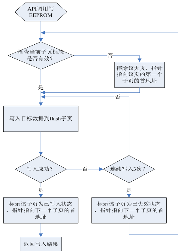
图五 写入模拟 EEPROM 数据流程
