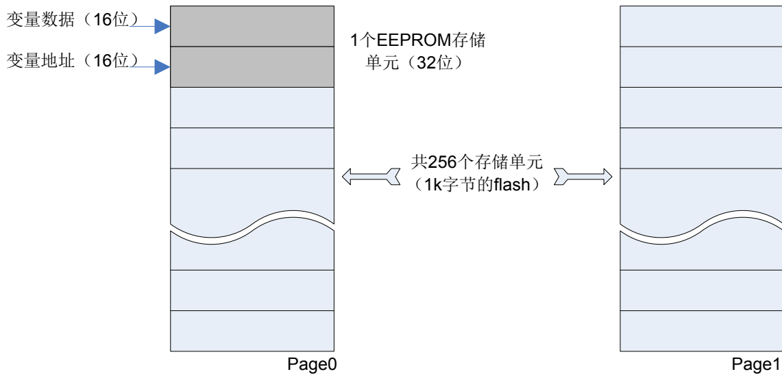
图二 EEPROM 存储单元格式
