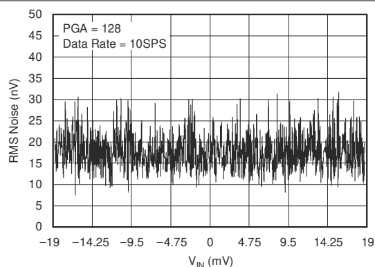
图 5-20. Noise vs Input Signal
