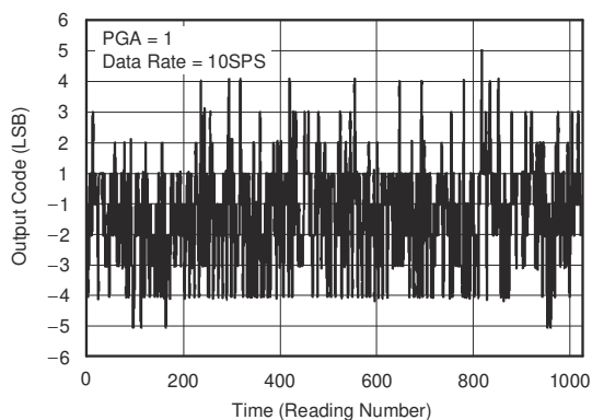
图 5-1. Noise Plot
