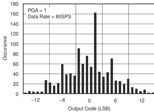
图 5-7. Noise Histogram
