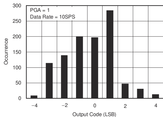
图 5-1. Noise Plot
