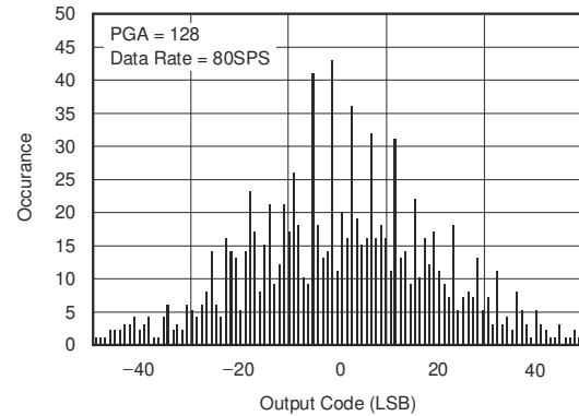
图 5-8. Noise Histogram
