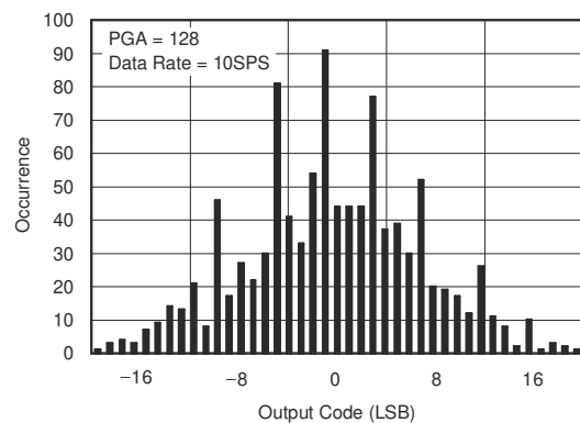
图 5-2. Noise Plot
