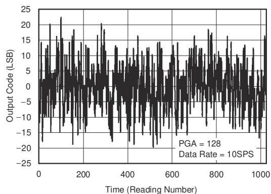
图 5-2. Noise Plot
