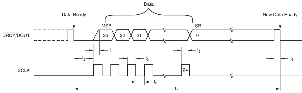
图 7-9. Data Retrieval Timing
