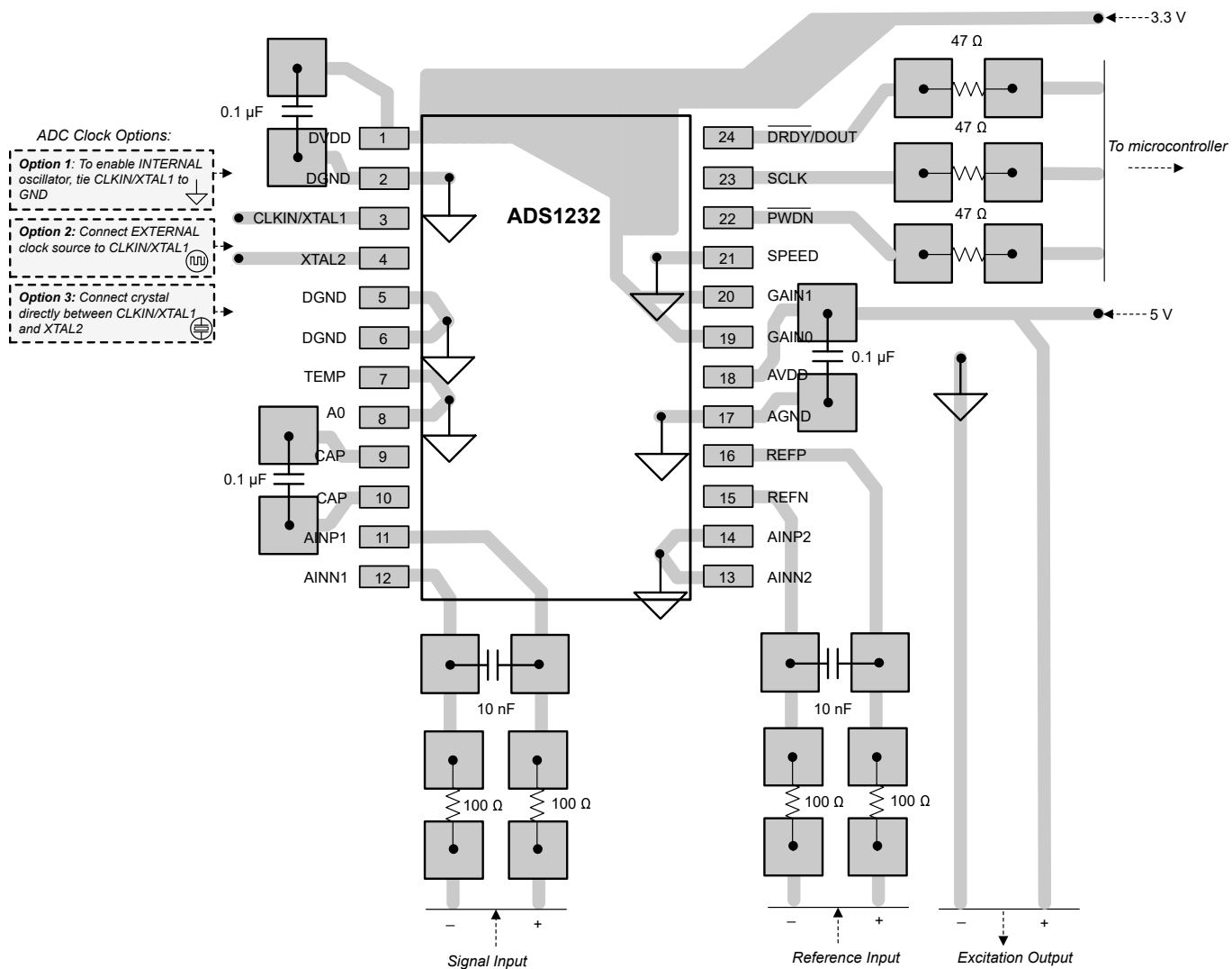
图 8-4. ADS1232 Layout Example
