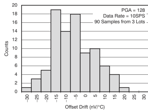
图 5-14. Offset Drift (25°C to 105°C)
