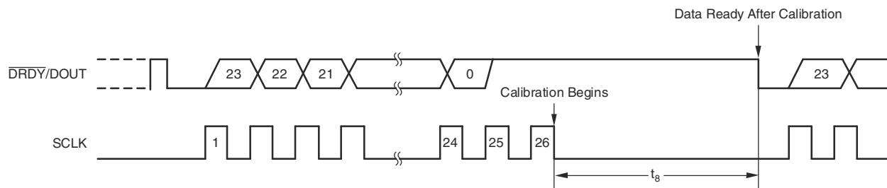
图 7-11. Offset-Calibration Timing
