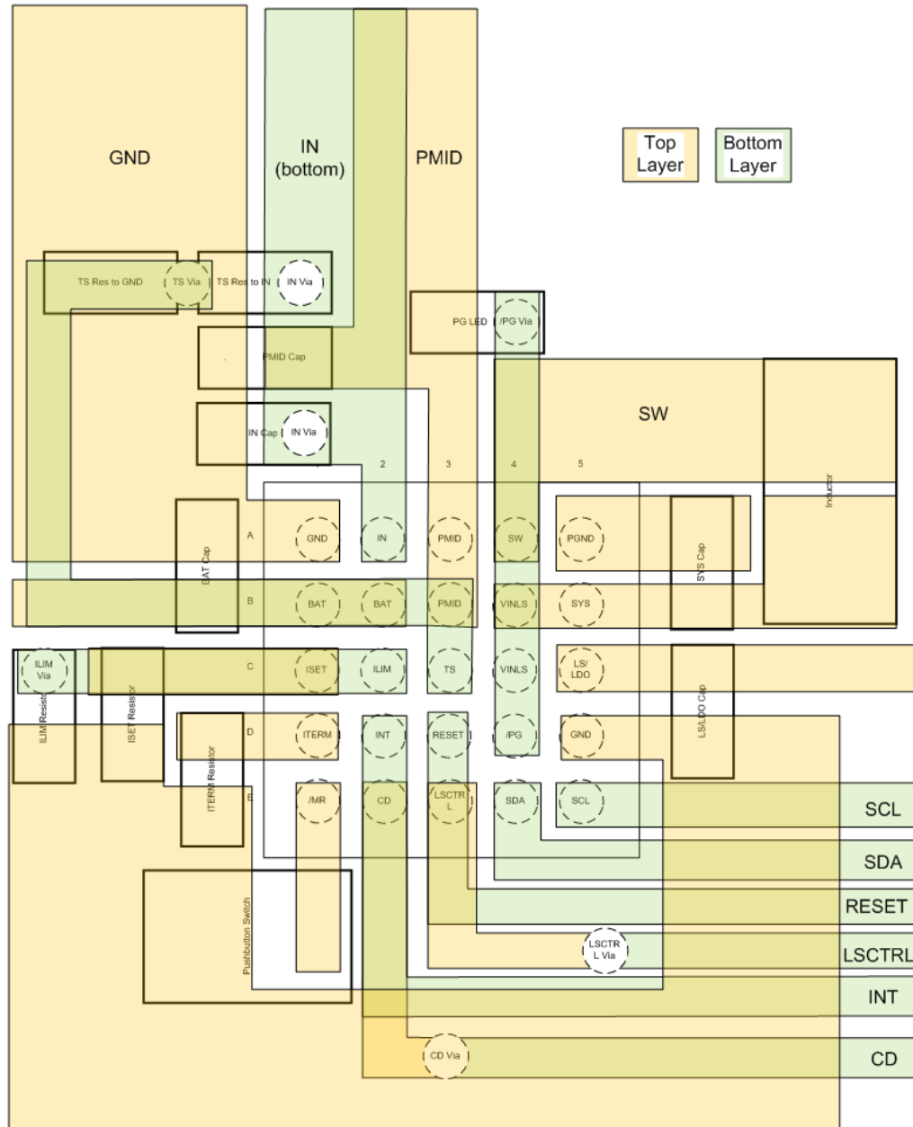
图 103. bq25120 Layout
