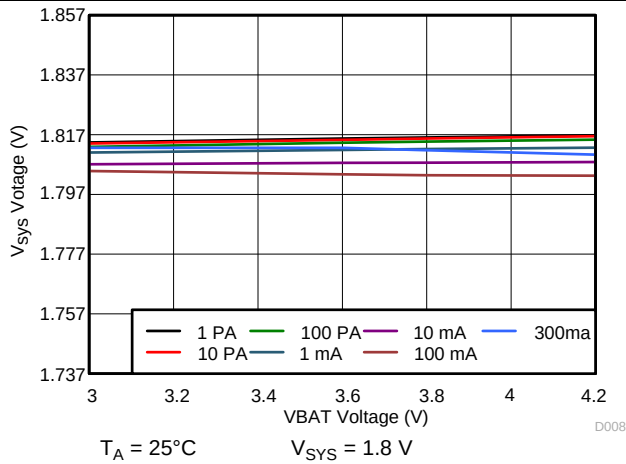
图 56. 1.8 V_{SYS} Line Regulation
