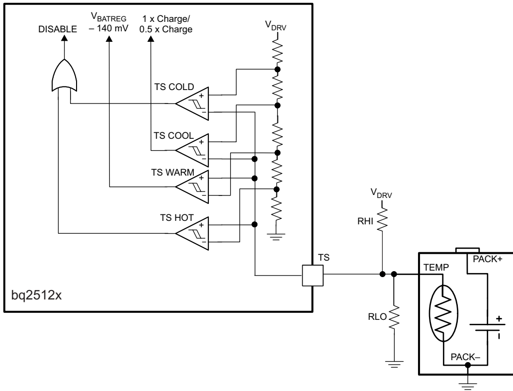
图 16. TS Circuit
