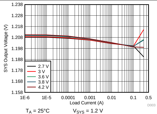
图 49. 1.2 V SYS Load Regulation
