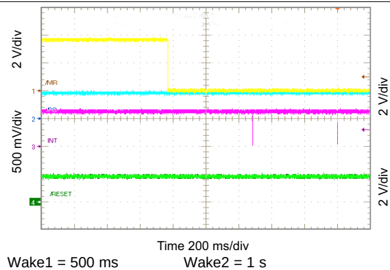
图 97. Show \overline{\text{MR}} Timing
