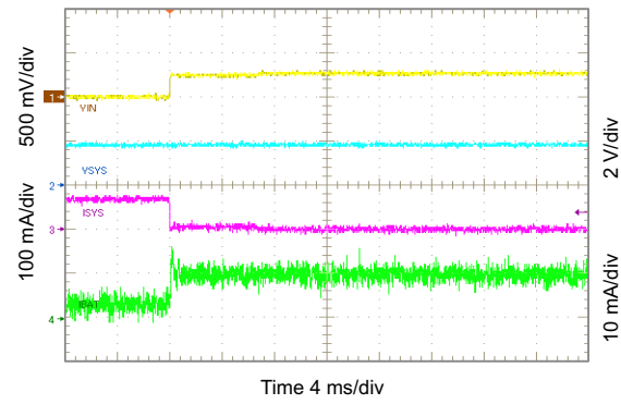
图 39. Exiting DPPM Mode
