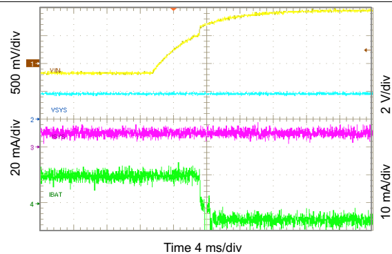
图 43. OVP Fault
