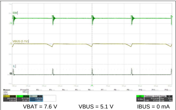
图 28. Buck Mode (OTG) PFM Switching
