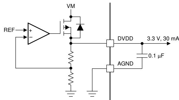
图 8-21. DVDD 线性稳压器方框图
