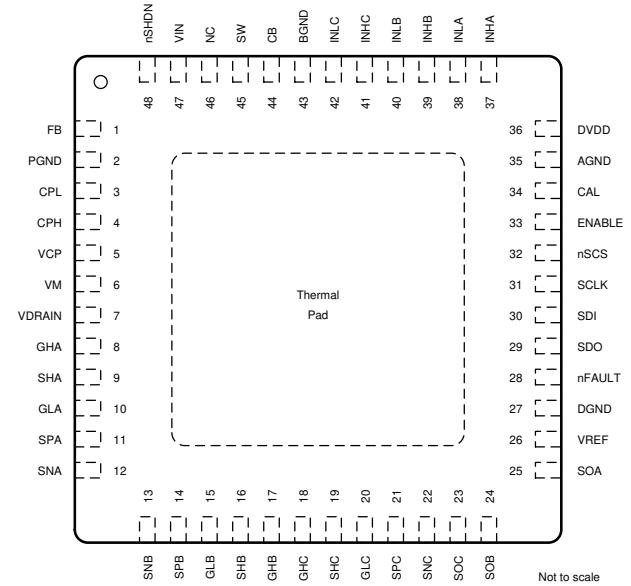
图 6-8. DRV8323RS RGZ 封装 48 引脚 VQFN ( 带有外露散热焊盘 ) 顶视图
