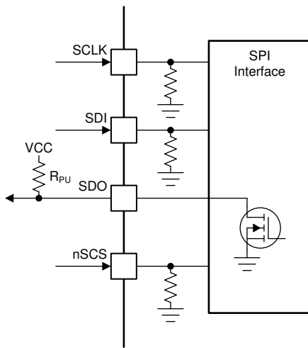
图 8-14. SPI
