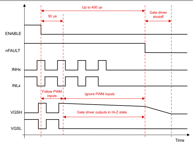
图 8-35. ENABLE 低电平时序图：ENABLE 引脚变为低电平后输入继续切换 50 μs
