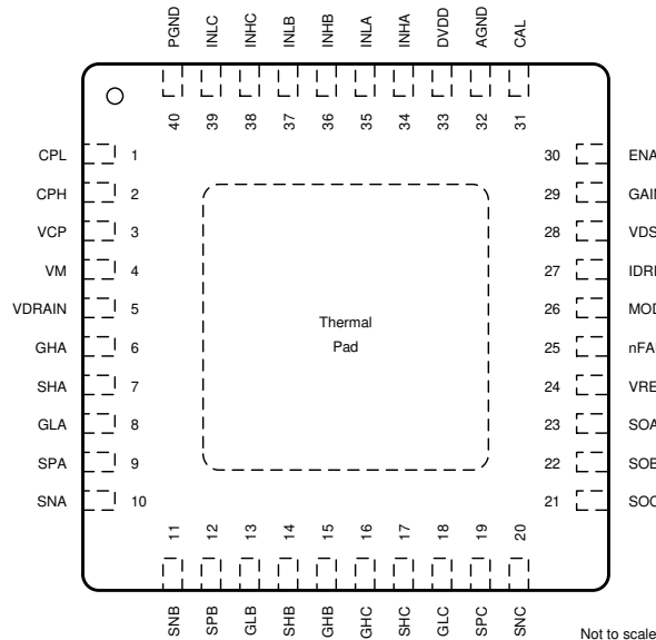
图 6-5. DRV8323H RTA 封装 40 引脚 WQFN (带有外露散热焊盘) 顶视图
