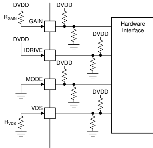
图 8-15. 硬件接口
